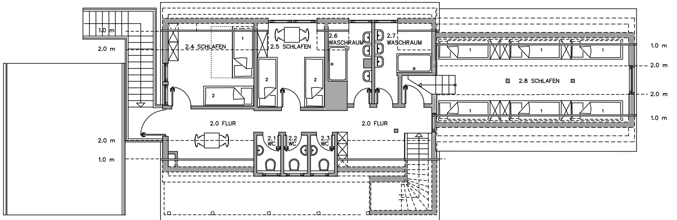
GRUNDRISS OBERGESCHOSS
