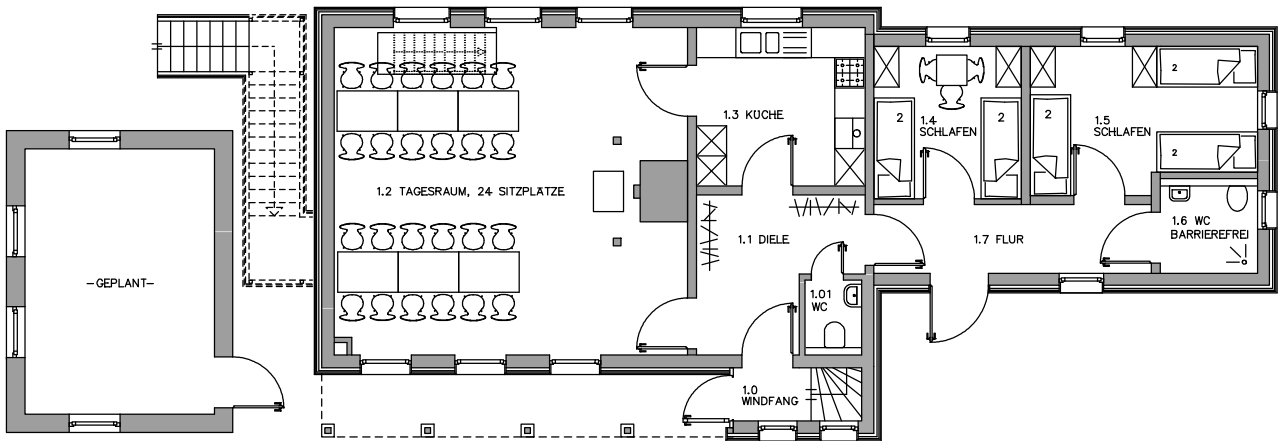
GRUNDRISS ERDGESCHOSS
