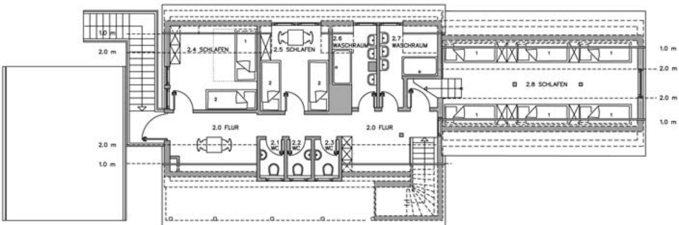
GRUNDRISS OBERGESCHOSS
