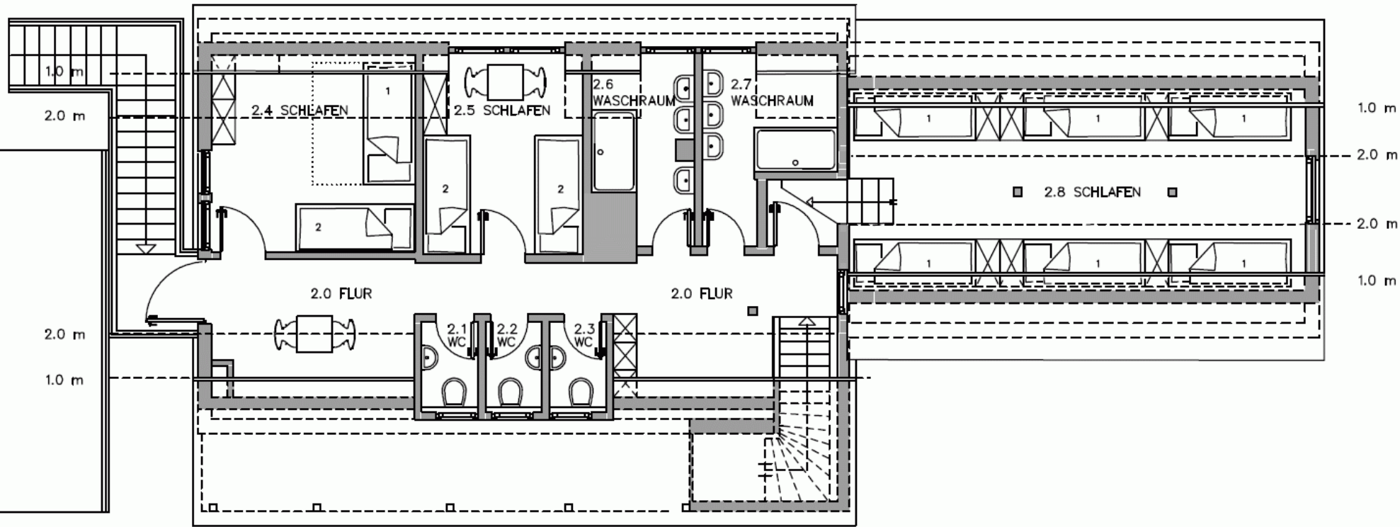
GRUNDRISS OBERGESCHOSS
